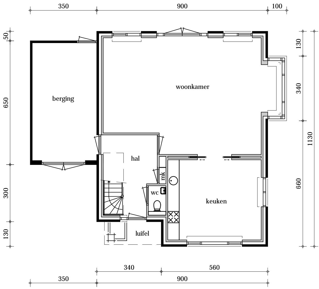
begane grond
